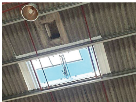
(Pose des lanterneaux Bluebac Pneu Reno par l'intérieure du bâtiment)
