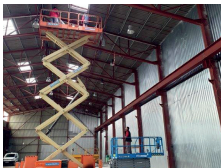
(Pose des lanterneaux Bluebac Pneu Reno par l'intérieure du bâtiment)
